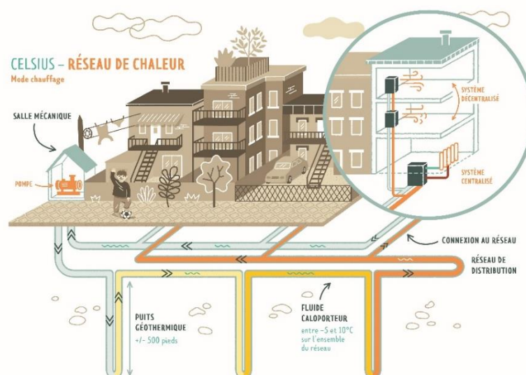
Figure 6 : Le réseau de chaleur CELSIUS en coupe illustré par Marie Levieil
